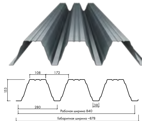
профнастил СТ150-840
