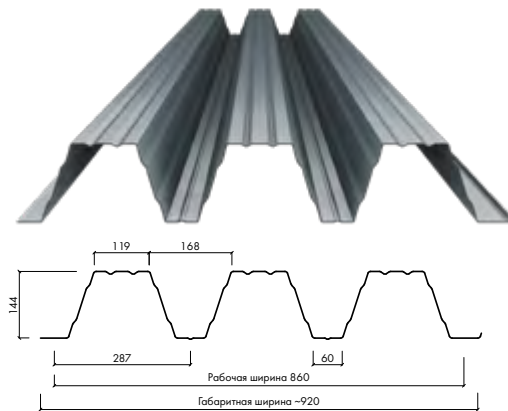
профнастил СТ144-860
