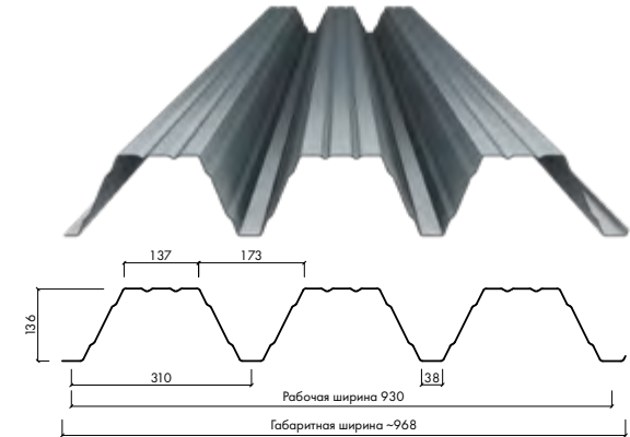
профнастил СТ135-930
