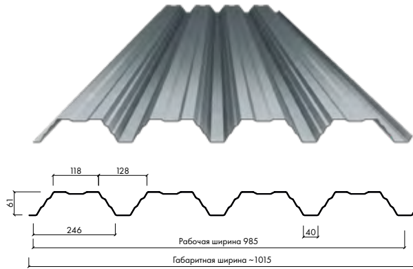
профнастил СТ62-985
