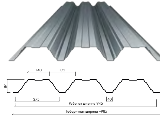
профнастил СТ90-945
