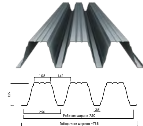
профнастил СТ160-750
